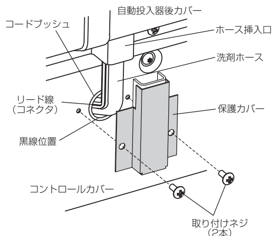
背面図
